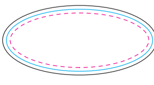
楕円形38.8×16.5mm (ゴルフマーカー クリップ部)
