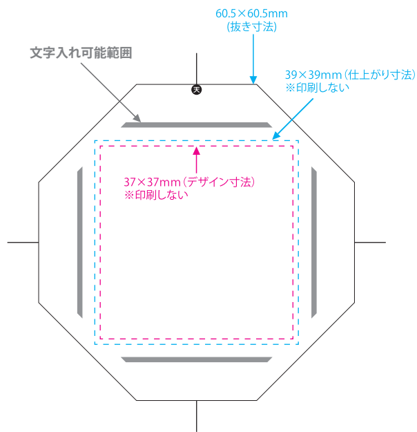
正方形 39×39mm
