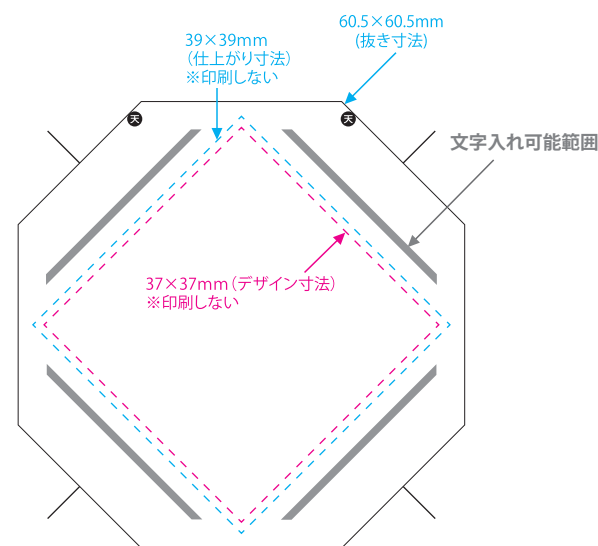
ひし形 39×39mm
