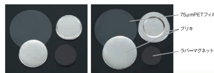
φ25、φ31、φ40mm用
