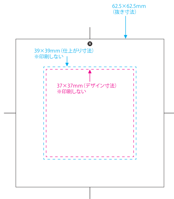
正方形 39×39mm
