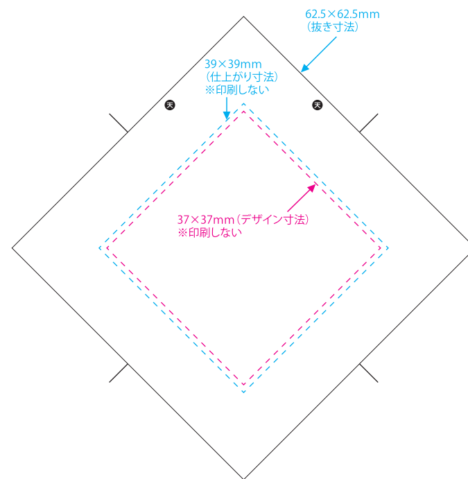
ひし形 39×39mm
